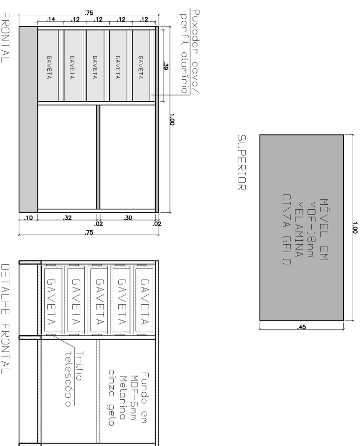
MÓVEL 5 GAVETAS E PRATELEIRAS 1.00 X 0.75 X 0.45
